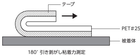
180°引き剥がし粘着力測定
