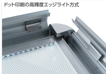
ドット印刷の高輝度エッジライト方式
