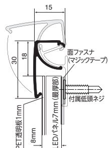
〈フレーム構造/断面〉
