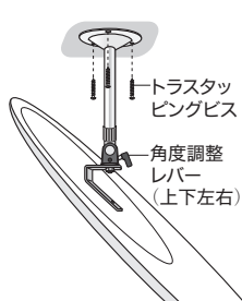
【COM-220の取付方法】
