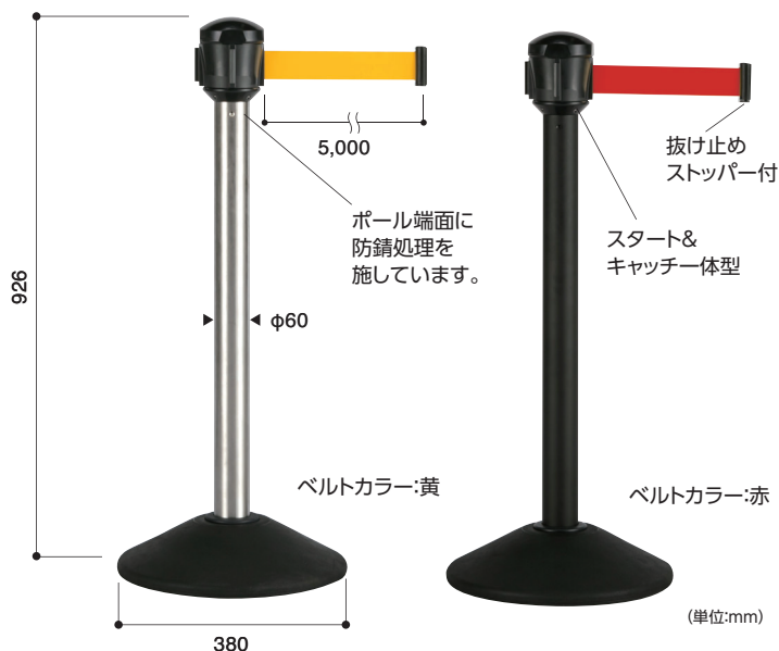
〈ステンレス ヘアライン〉
