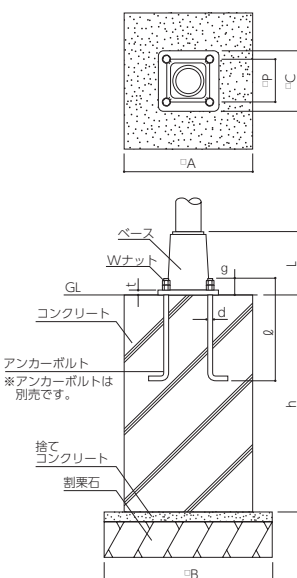
φ 140 用 (ポール高 6m ～ 10m)
