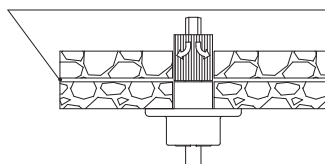
天井ボードの2枚張り
