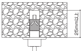
木材・スラブ等使用時の孔の深さ
