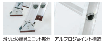
滑り止め端ユニット部分 アルフロジョイント構造
