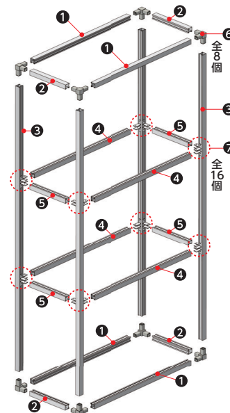
■展開図 製作使用例 W600mm×D200mm×H1,800mm
