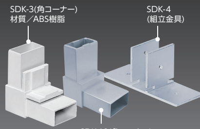
SDK-10(角コーナー) 材質/アルミ
