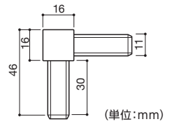
ジョイント16寸法
