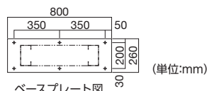
ベースプレート図
