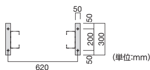
ベースアングル図
