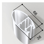
エッグ支柱（単位:mm）
