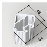
キューブ支柱（単位:mm）
