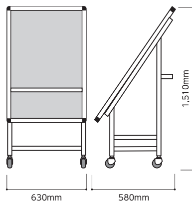
■ 材 質: 本体アルミ押出し材/アルマイト ■ 上部ポスターサイズ: A1 (594mm×841mm) ■ 有効表示寸法: W580mm×H827mm ■ 総重量: 約18kg(パネル含) ■ 耐荷重: 100kg
