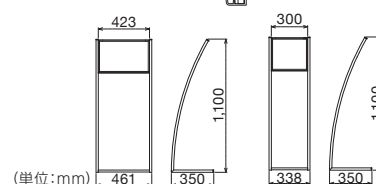
上部よりスライドセット
