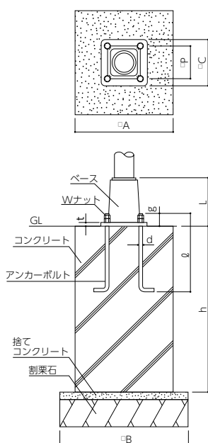
φ 100 用 ※アンカーボルトは付属していません。
