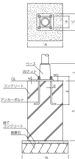
φ 140 用 ※アンカーボルトは付属していません。
