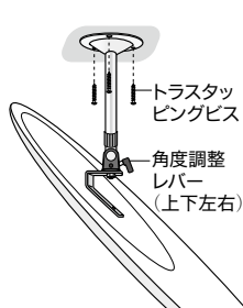
【COM-220の取付方法】
