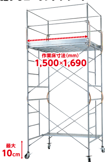
アウトリガー取付側
