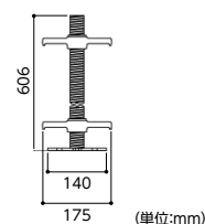
ジャッキベース
