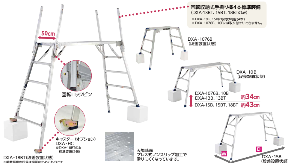
DXA-18BT (段差設置状態) ※掲載写真の段差は撮影のためのものです
