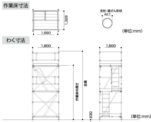
ゆとりのスペース&開閉式作業床
