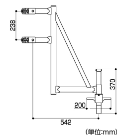
アウトリガー
