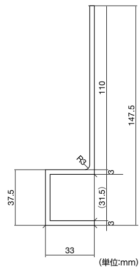
〈断面図〉
