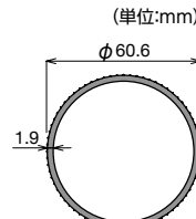
SAS-260 (補助柱)
