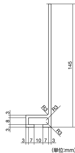
〈断面図〉
