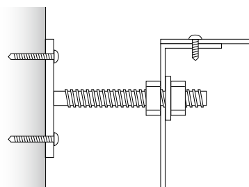
取付図
