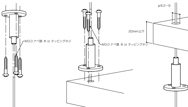
天井、壁などへ取り付ける場合
