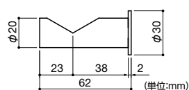
■真チュウ+ウレタン／A4×30
