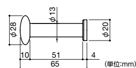
■真チュウ+ウレタン／A4×30
