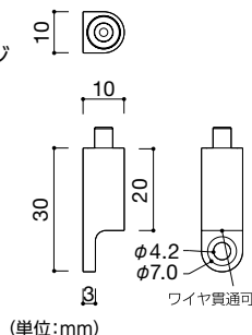
パネルなどを側面で吊る場合
