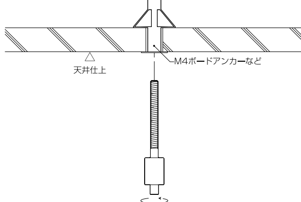
天井へ取り付ける場合
