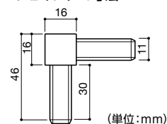
ジョイント16寸法
