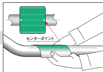
③巻き付ける 手すりの頂点と標示板のセンターポイントを合わせ、手すりになじませながら巻き付ける。
