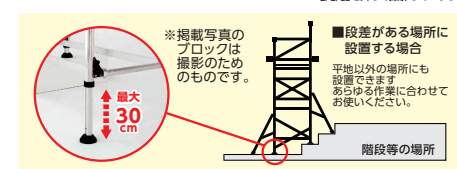
アウトリガー 開閉式建柱 開閉式作業床
