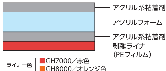
〈テープ構造〉
