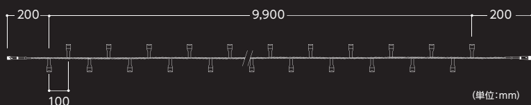
2芯パワーコード Ver.2 ブラックコード (単位:mm)
