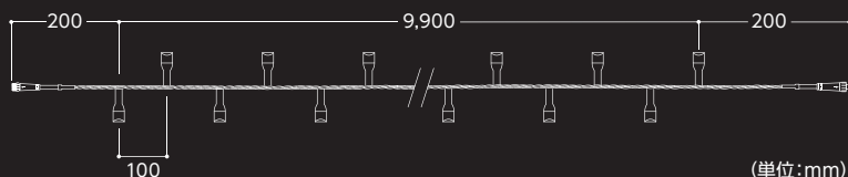
2芯パワーコード Ver.2 ブラックコード (単位:mm)
