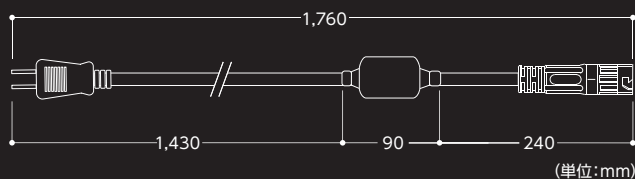
2芯ハイグレード専用 パワーコード
